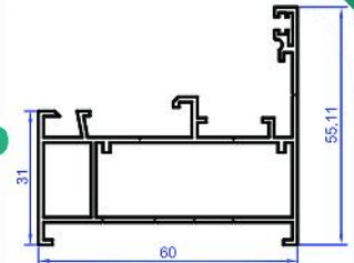
فریم Frame AK.H601 1.22kg/m
