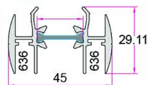
پروفیل وسط چهار لنگه Adjoining Sash Adapter 0.892Kg/m
