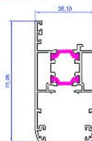
لنگه زهوارخور یراق UPVC Sliding Sash 1.125Kg/m
