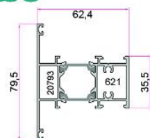
وادر لیفت اند اسلاید Tripetalous Profile 1.550Kg/m
