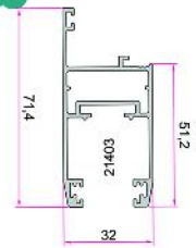
لنگه زهوار خور Sash 0.885Kg/m
