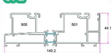
چهار چوب دو ریل لیفت اند اسلاید Lift and Slide Frame 3.035Kg/m
