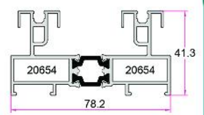
چهارچوب کشویی بدون ریل توری Sliding Frame 1.580Kg/m
