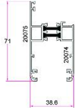
لنگه زهوار خور Sliding Sash 1.060Kg/m
