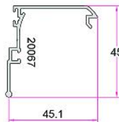
درپوش Cap 0.417Kg/m
