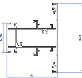
وادار Mullion AK.H604 1.3kg/m
