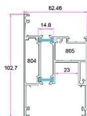
لنگه لیفت اند اسلاید Lift and Slide Sash 2.357Kg/m
