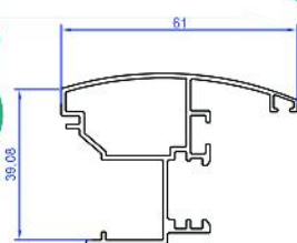
وادار Mullion AK.H614 0.967Kg/m
