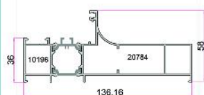
کتیبه لیفت اند اسلاید مونوریل سری ۱۳۶ و ۱۴۰ Engraving Profile 1.750Kg/m
