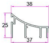
درپوش ریل Rail Cover 0.450Kg/m
