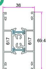
وادر بدون زهوار Tripetalus 1.278Kg/m
