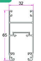
لنگه کشویی ساده کبپر دار Simple Sliding Sash 0.860Kg/m
