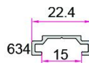
پروفیل جای تسمه Strap Holder 0.183Kg/m
