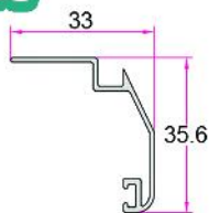
روکوب اختصاصی ۳ سانتیمتری Casing 0.220Kg/m
