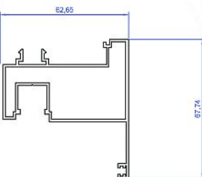
دولنگه لولایی Middle Sash AK.H606 1.1kg/m
