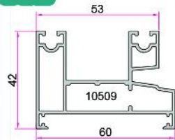
فریم Frame 1.022Kg/m
