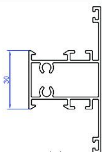
وادار Mullion AK.H614 0.967Kg/m
