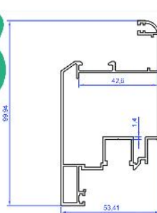
لنگه درب Sash Door AK.H617 1.24Kg/m
