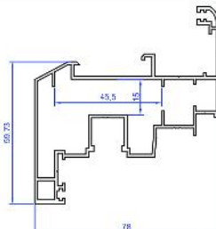
لنگه پنجره Win Sash AK.H602 1.4kg/m
