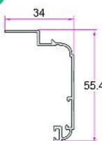
روکوب اختصاصی ۵ سانتیمتری Casing 0.360Kg/m
