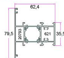
وادار لیفت اند اسلاید Tripetalous Profile 1.550Kg/m
