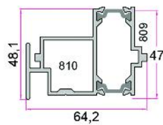
چهار لنگه لیفت اند اسلاید The Middle Four Vent 1.600Kg/m
