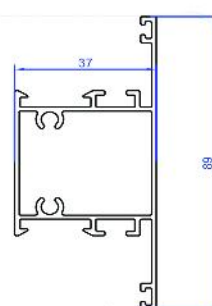
وادار Mullion AK.H615 0.88Kg/m
