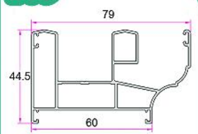
چهار چوب کشویی طرح دار Sliding Frame 1.060Kg/m
