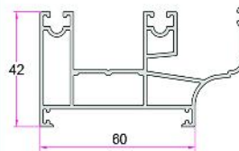
فریم Frame 1.280Kg/m
