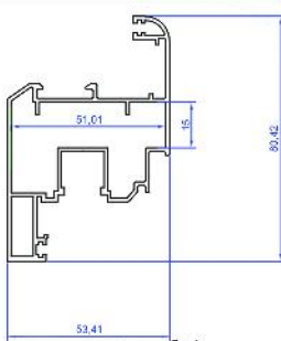
لنگه پنجره Win Sash AK.H612 1.13Kg/m
