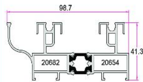
چهارچوب کشویی با ریل توری Sliding Fram With Fly Screen Rail 1.540Kg/m
