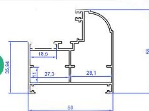
فریم Frame AK.H611 1.05Kg/m
