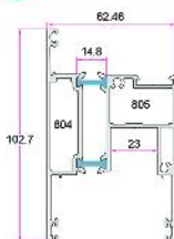
لنگه لیفت اند اسلاید Lift and Slide Sash 2.537Kg/m
