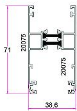
لنگه بدون زهوار Sliding Sash 1.180Kg/m
