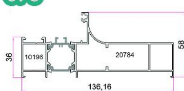
کتیبه لیفت اند اسلاید مونوریل سری ۱۳۶ و ۱۴۰ Engraving Profile 1.750Kg/m
