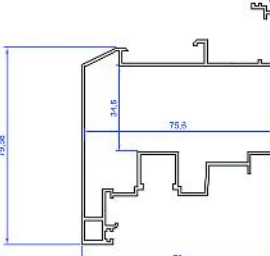
لنگه درب Sash Door AK.H605 1.6kg/m
