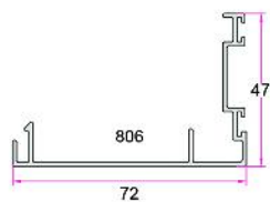
مکمل لنگه Cap 0.650Kg/m
