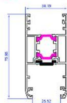
لنگه بدون زهوار یراق UPVC خور Sliding Sash 1.115Kg/m
