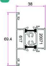
وادار زهوار خور Tripetalus 1.102Kg/m
